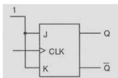
T-FF
