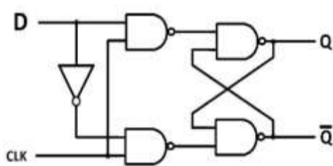
D-FF
