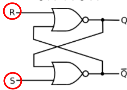
SR-NOR
